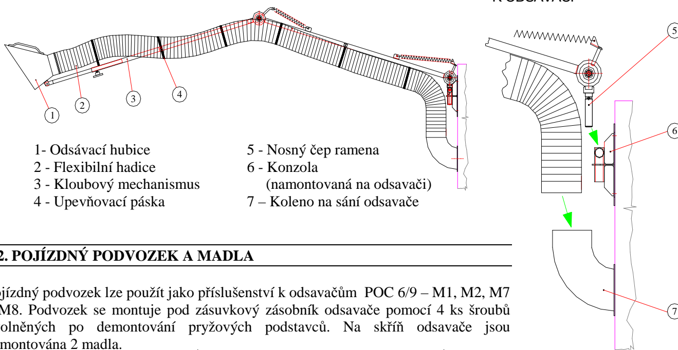
DETAIL PŘIPOJENÍ RAMENA K ODSAVAČI
