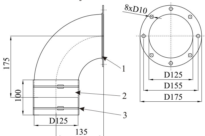
Obr. 3 Koleno D125-obj.č.430260
